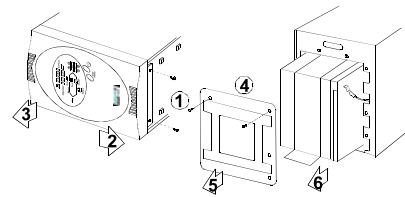
Abb. 4: ZINTO D-Serie
